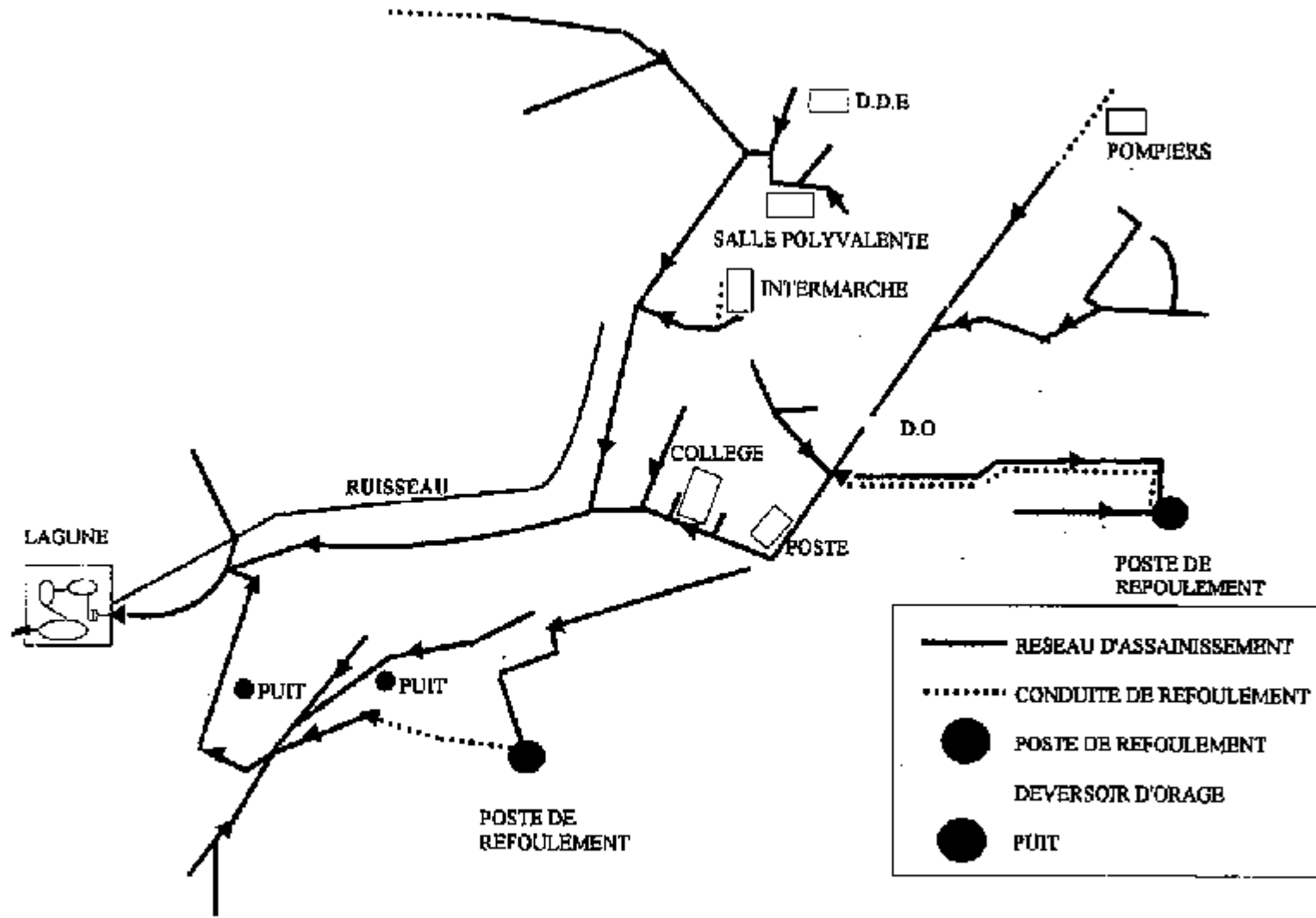
Fig. 2-b : synoptique du réseau d'assainissement de Soumbergon
